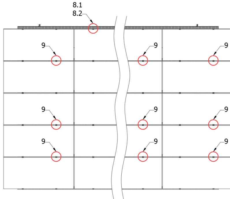
Rys. 4 Widok konstrukcji od góry
