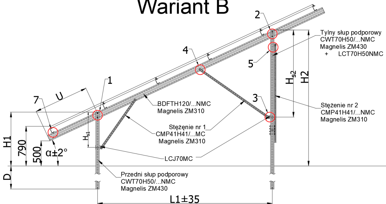
Rys. 1 Widok boczny konstrukcji
