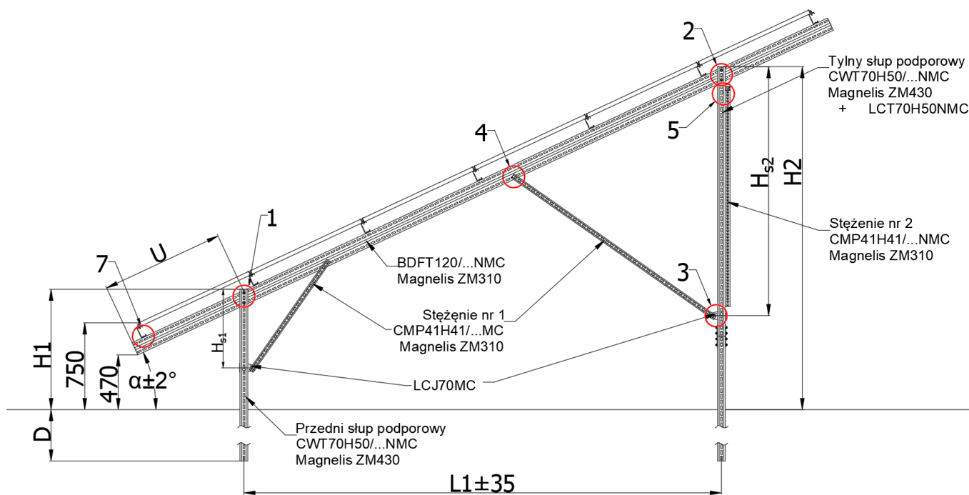
Rys. 1 Widok boczny konstrukcji
