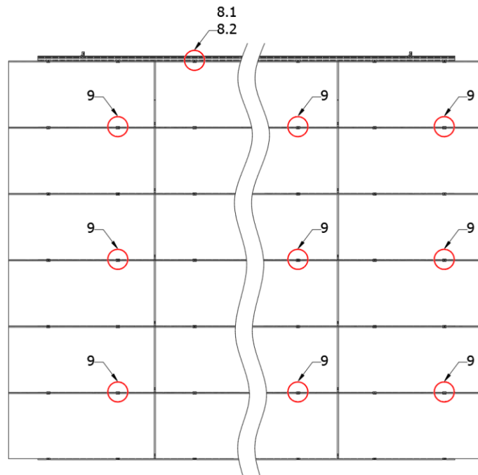
Rys. 4 Widok konstrukcji od góry
