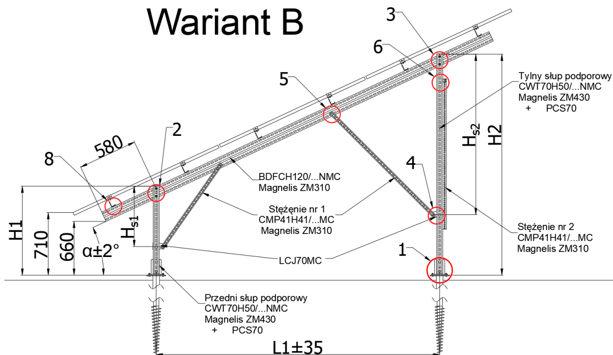
Rys. 1 Widok boczny konstrukcji
